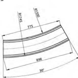
Römertreppensegment 6-teilig 30° Ri = 1500 mm
