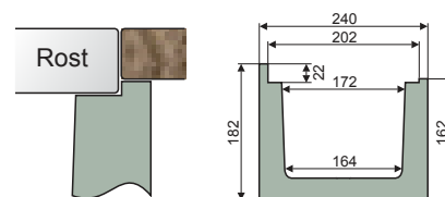
Rinnenhinterkante wird mit Fliesen oder Steinplatten abgedeckt
