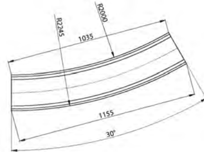
Römertreppensegment 6-teilig 30° Ri = 2000 mm
