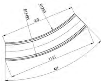
Römertreppensegment 4-teilig 45° Ri = 1250 m m
