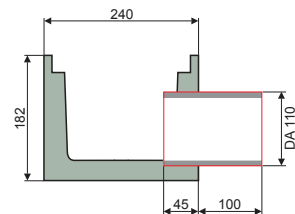
Schnitt seitlicher Ablauf DN-100
