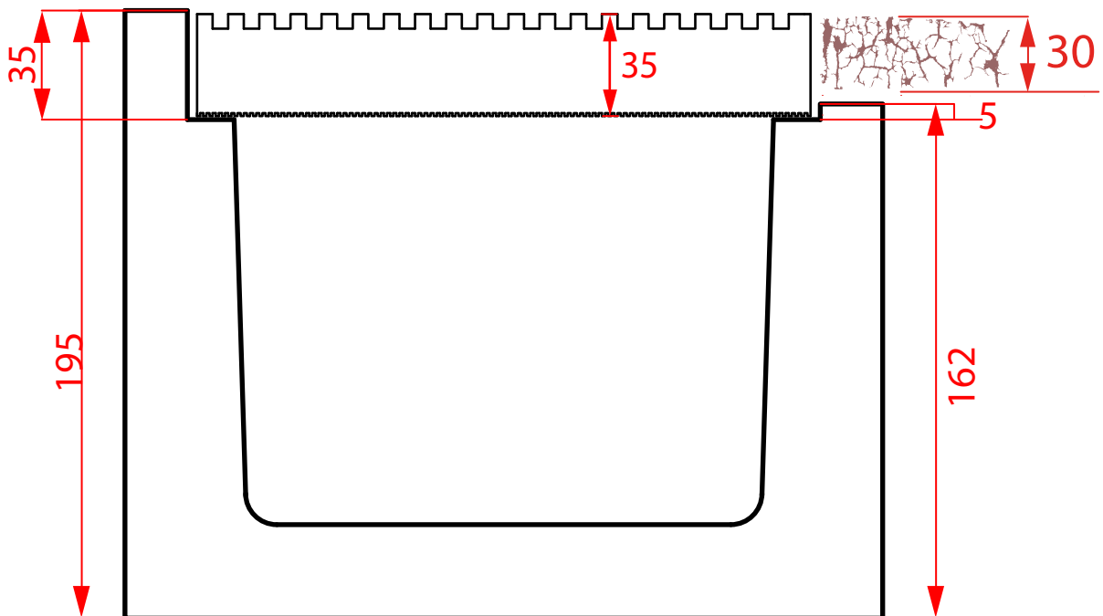
Hallenbad 195 x 162 mm (Rost 35 mm) für Plattenverlegung ca. 35 - 40 mm
