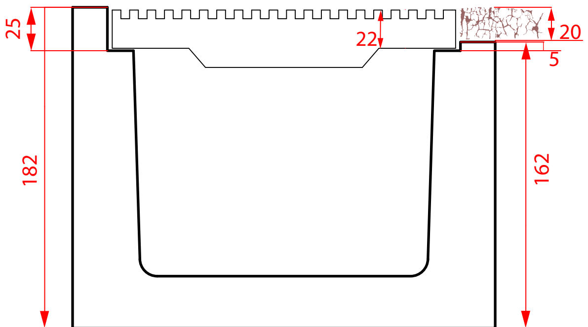
Hallenbad = 182 x 162 mm (Rost 22 mm)
