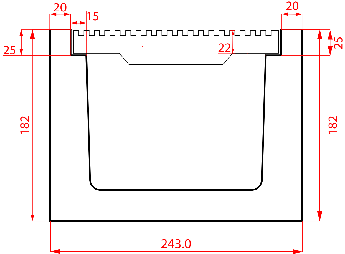
Freibecken = Standard 182 x 182 mm (Rost 22 mm)
